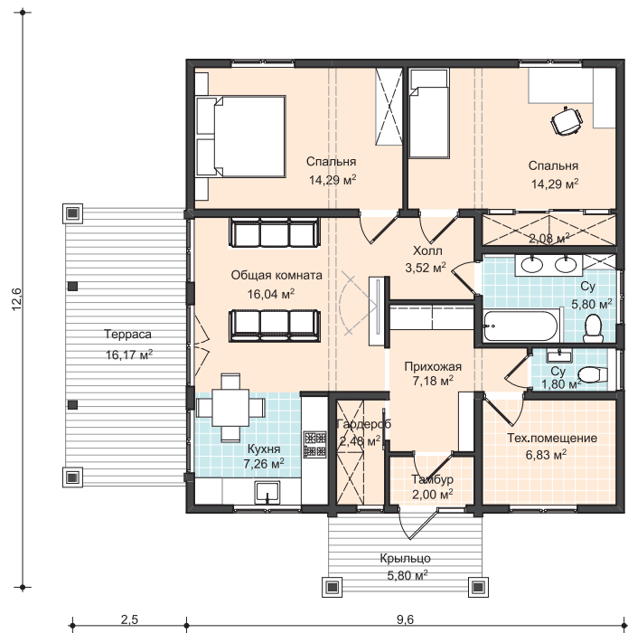
План 1 этажа масштаб 1:150
