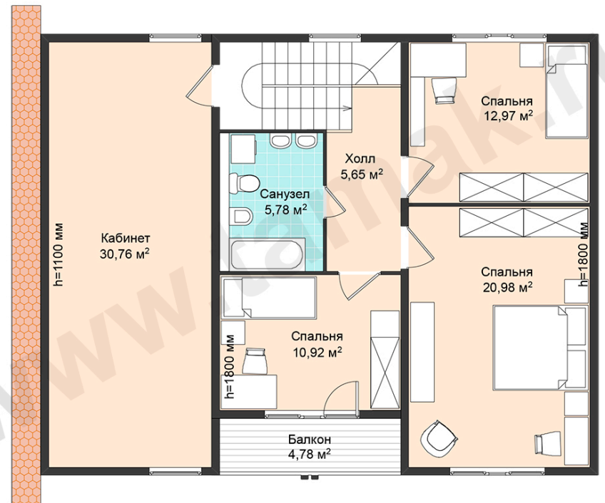
План 2 этажа
