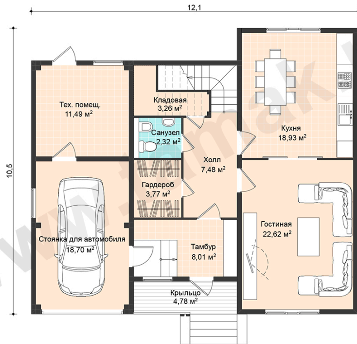
План 1 этажа
